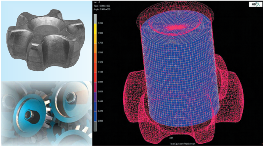
Bild 15: Simulation in der Umformtechnik (Video)
